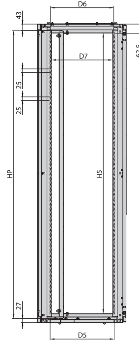
A-A section
