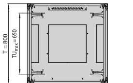
Schnitt D-D (Schrantiefe 800 mm)
