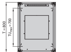
Schnitt C-C (Schrantiefe 800 mm)
