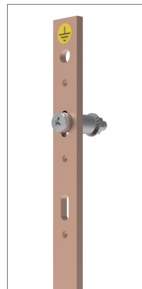
Vertikale Erdungsschiene für Befestigung an Tiefenstreben
