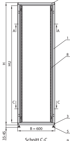
Schnitt C-C (Schrantiefe 600 mm)
