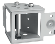
Nivellierschraube für den Sockel zum Schrank SZB IT oder DSR IT
