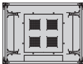
Schnitt B-B (Schrantiefe 600 mm)
