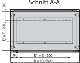
Schnitt A-A
