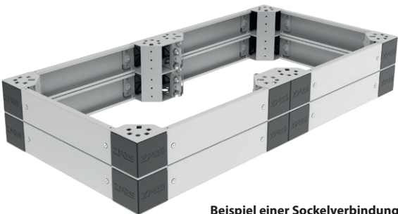
Beispiel einer Sockelverbindung
