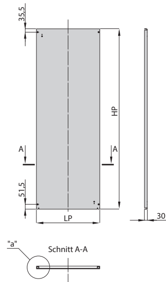
Montageplatte
