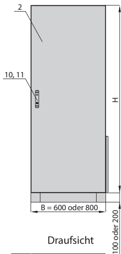
Vorderansicht (Schränk mit einfügiger Tür)
