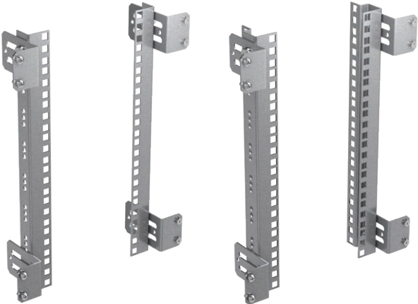
Gestell aus 19"-Tragwinkeln
