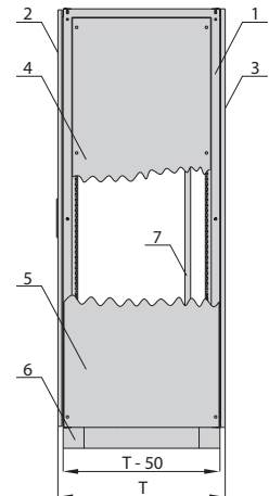
Seitenansicht (Vergleichung der ebene und herausstehende Seitenwand)
