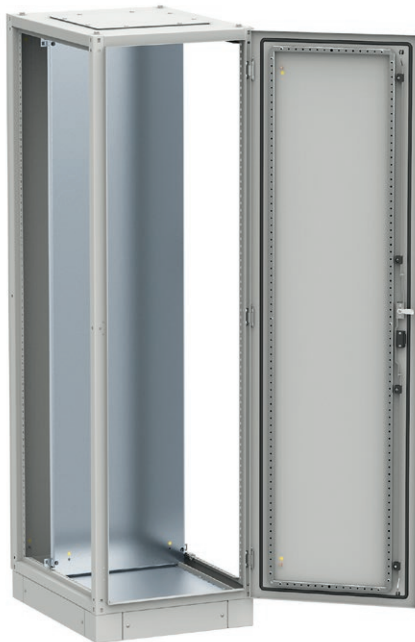
Schaltschrank 600 mm breit ohne Seitenwände, vorgesehen zur Anreihung
