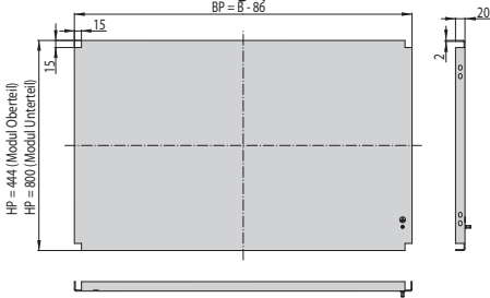
Montageplatte
