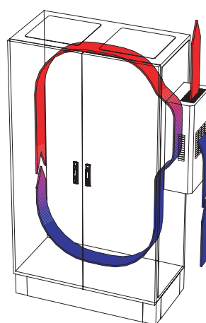
Wandbau-Kühlgerät
