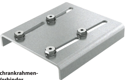
Schrankrahmen- -Verbinder Typ A
