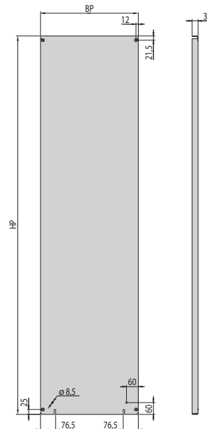
Montageplatte
