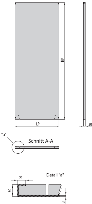
Montageplatte
