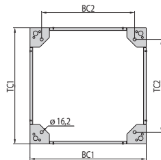
Sockel verschraubt (Abstand der Befestigungslöchungen)
