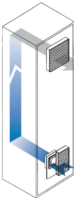
Beispiel der Luftführung in einem Schrank durch Einsatz eines Filterlüfters und eines Austrittsfilters
