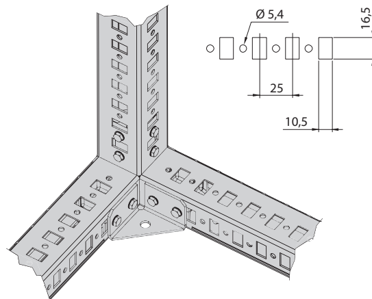
Realisierung von Öffnungen im Schrankrahmen SZE3: - Öffnungen 10,5 x 16,5 mm für Käfigmuttern M8 mit Flügeln, - Öffnungen Ø 5,4 mm für selbstformende Schrauben M6
