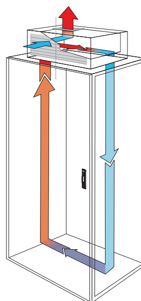
Dach-Kühlgerät
