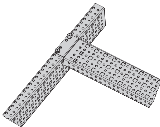
Beispielhafte Verbindung der Montageschienen Typ A und B mithilfe der selbstformenden Schrauben M6
