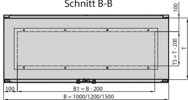
Schnitt B-B
