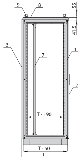
Vorderansicht (mit Dach und Transportösen)
