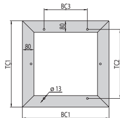
Sockel geschweisst (Abstand der Befestigungslöchungen)
