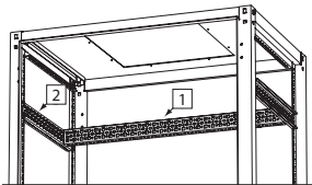
1. Montageschiene CLASSIC 2. Querträger CLASSIC
