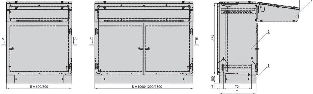
Schnitt A-A
