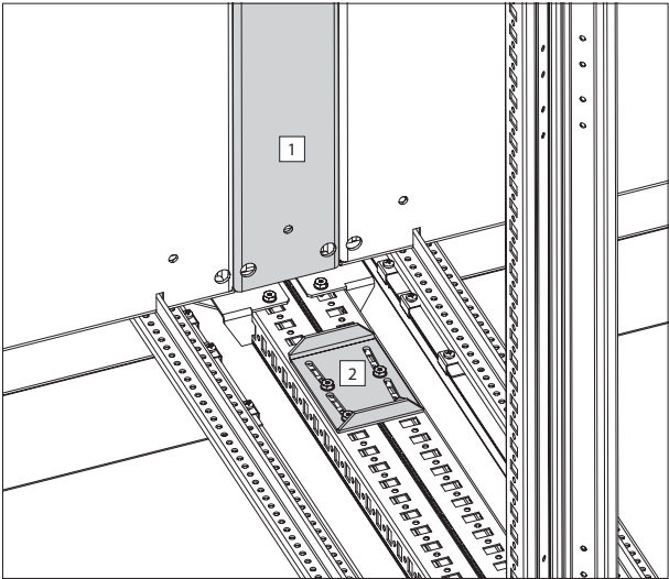
1 - Verbinder für Montageplatten 2 - Schrankrahmen-Verbinder - Typ A
