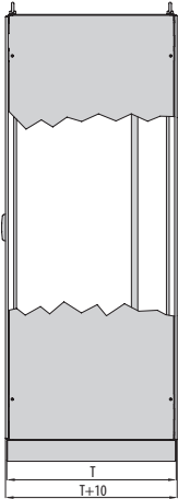
Seitenansicht (Schrank mit Seitenwand)
