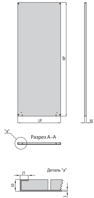
Монтажная панель
