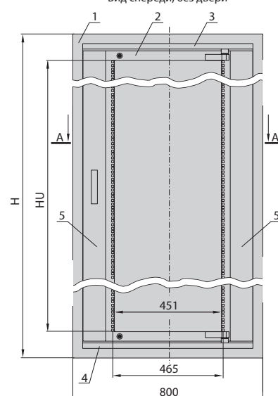
Шкаф с поворотной рамой
