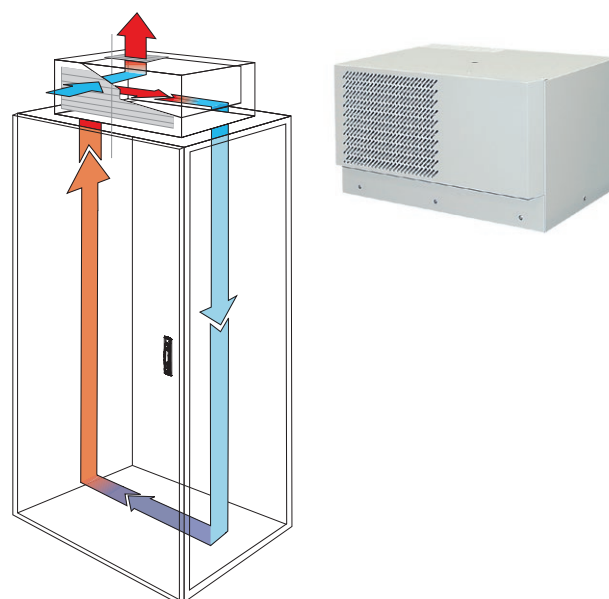
Вариант кондиционера, устанавливаемого на крыше шкафа
