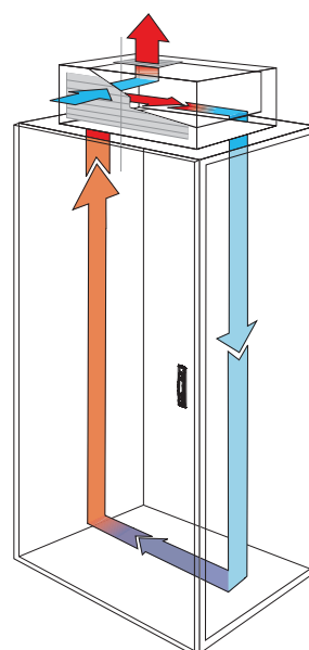
Вариант кондиционера, устанавливаемого на крыше шкафа
