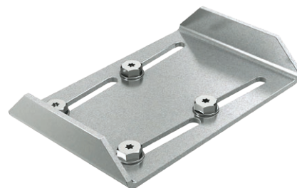
Соединитель каркаса – тип А
