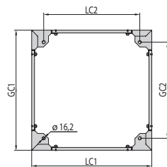
Цоколь сборный (отверстия для анкеровки)
