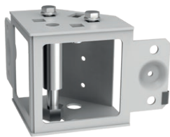
Уголок цоколя с винтом, регулирующим высоту
