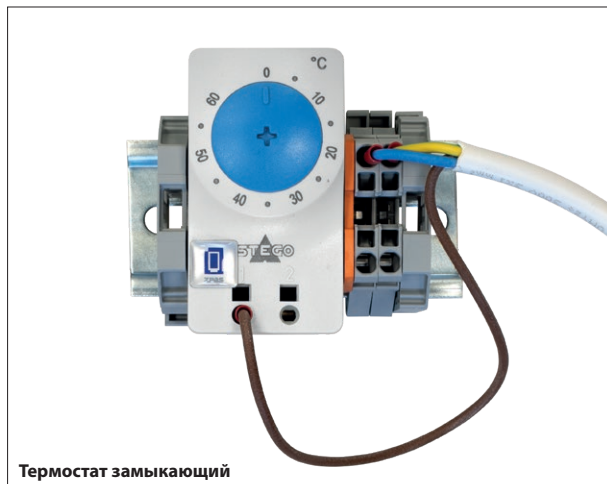
Термостат замыкающий
