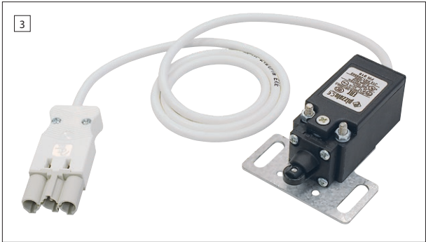
Комплект концевого выключателя для шкафа SZE3
