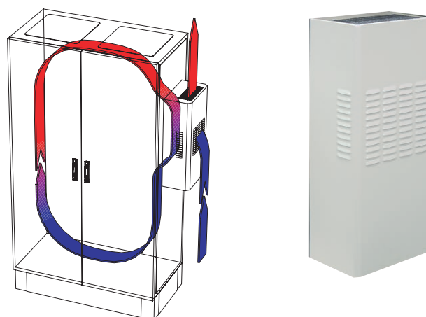
Пример установки кондиционера на боковой стенке шкафа
