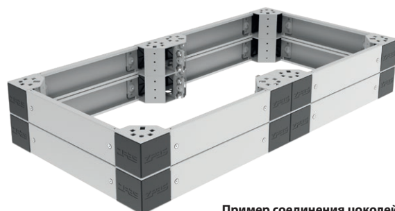
Пример соединения цоколей
