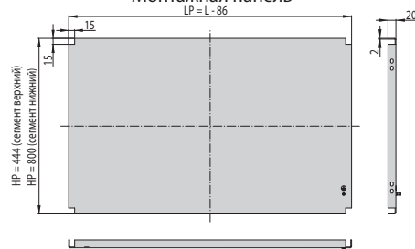
Монтажная панель
