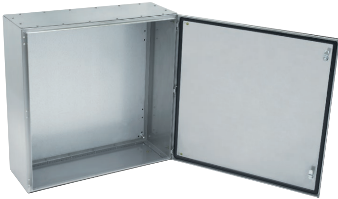
Шкаф SWN Inox размером 800 x 800 x 300 мм, партномер: WZ-SWN-808030-N1-000, две заглушки (нижняя и верхняя)
