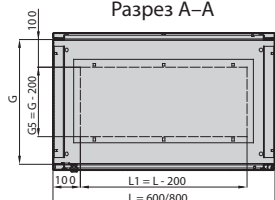
Разрез А-А
