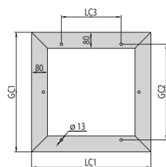
Цоколь сварной (отверстия для анкеровки)
