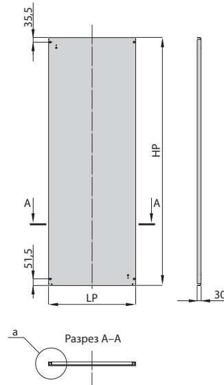
Монтажная панель
