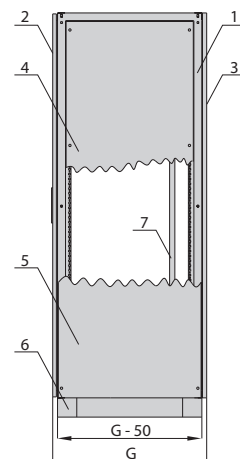
Вид с боку (сравнение вкладной и выступающей боковых стенок)
