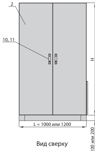
Вид спереди (шкаф с двустворчатой дверью)
