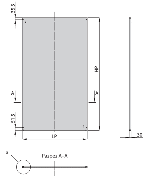
Монтажная панель
